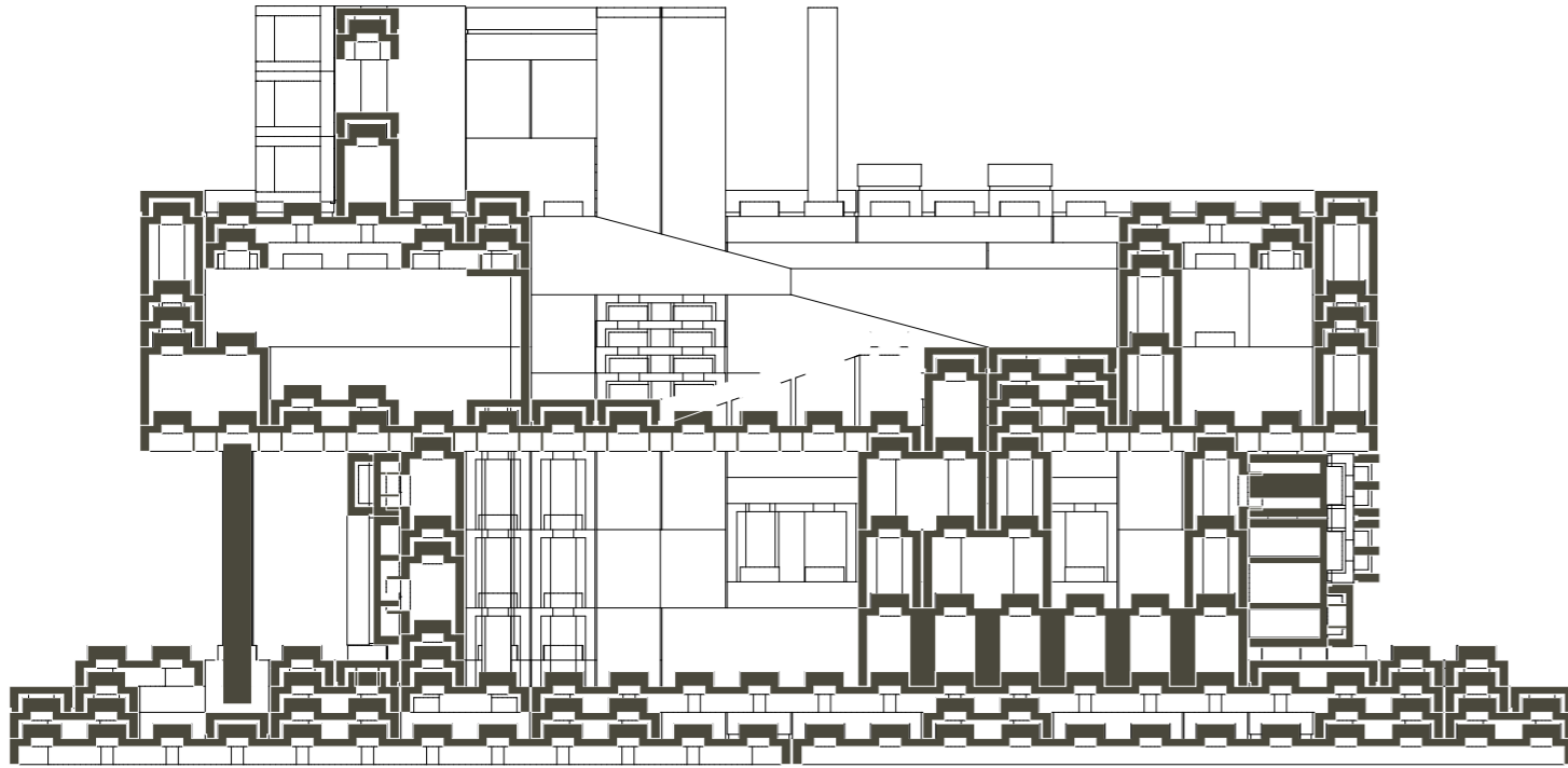
Section A-A
