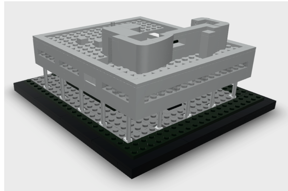
Autodesk A360
